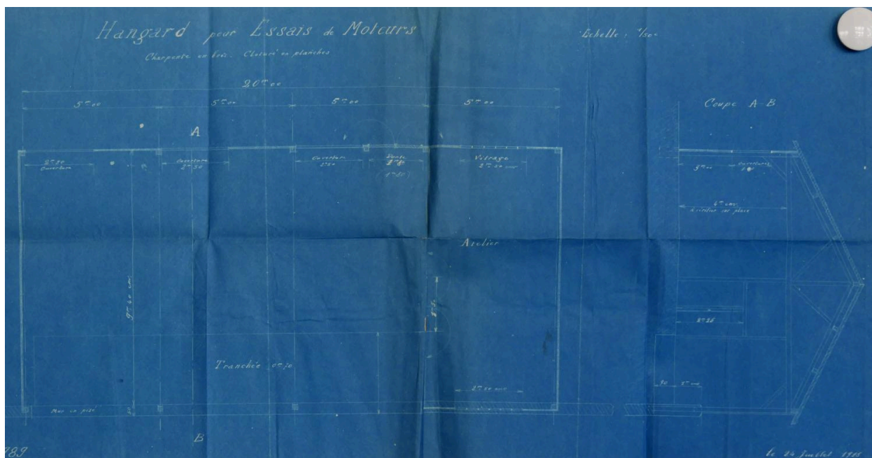
Hangar pour essais de moteurs, charpente 1918 (AC Lyon 314W/595)
