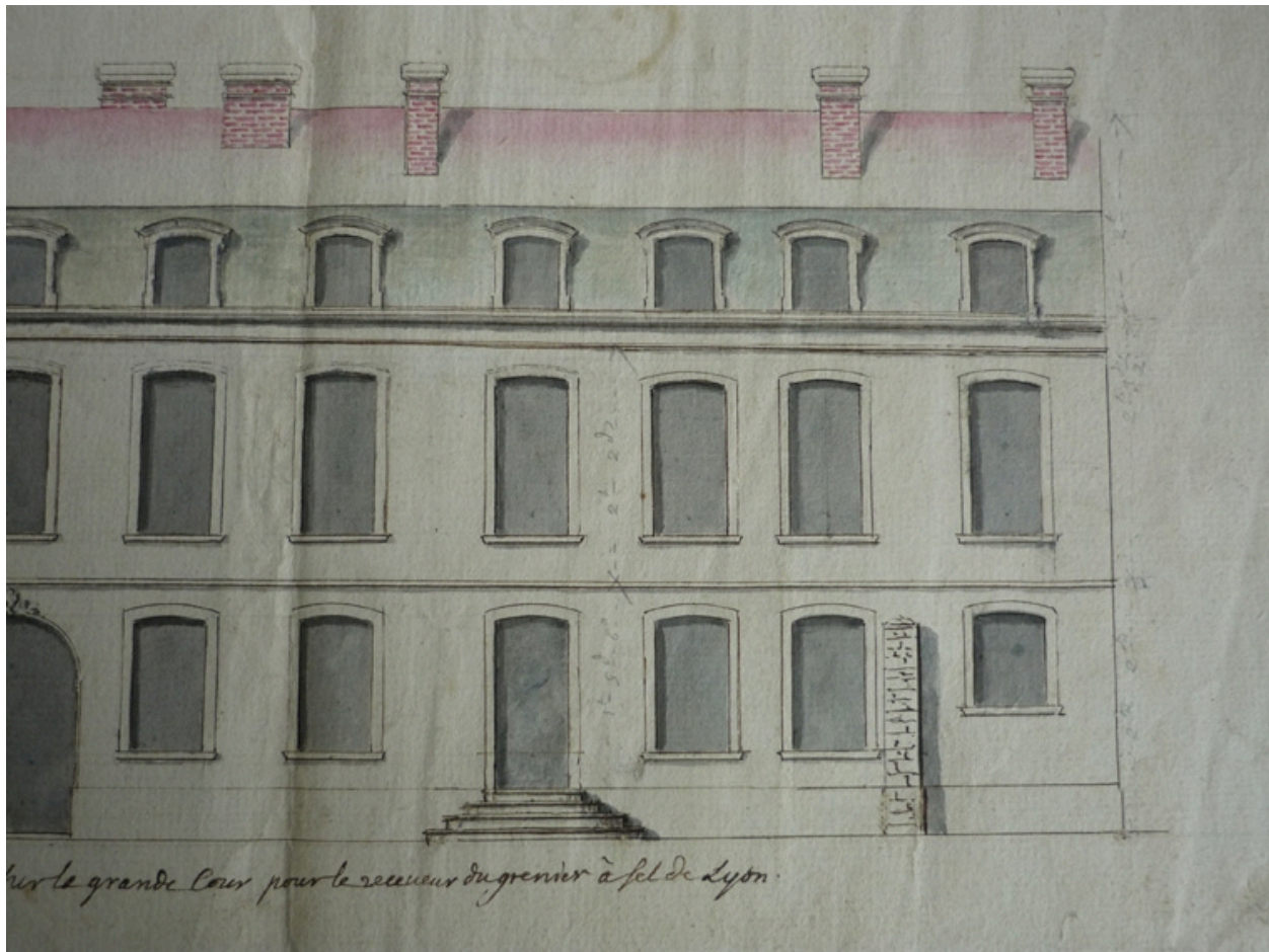
Élévation d'un corps de logis pour le receveur du grenier à sel, 1740 (détail du bâtiment : partie de droite). Plan AC Lyon. Fonds des HCL ; B422
