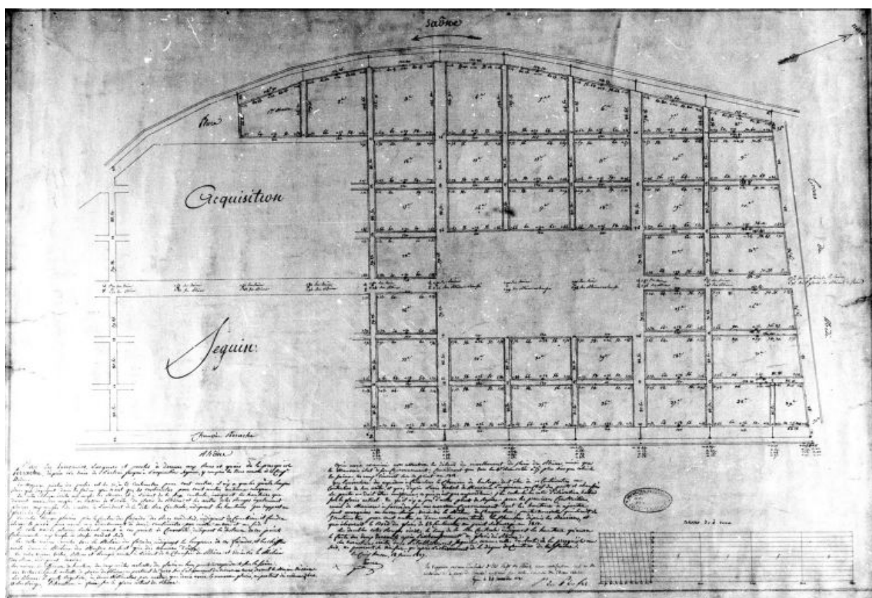
Plan des longueurs, largeurs et pentes à donner aux rues, quais de la presqu'île Perrache... / Jean-François Terrat, 18 juin 1827 (AC Lyon : 0002 S 0236 2)
