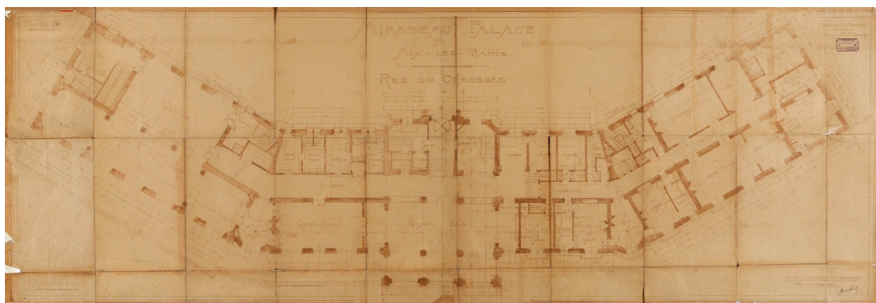
Plan du rez-de-chaussée, 1908
