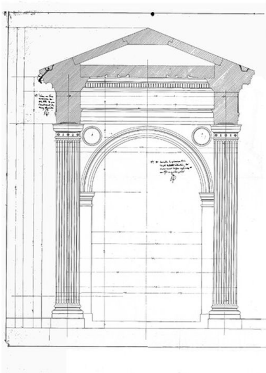
Chapelle de l'Observance, coupe du porche
