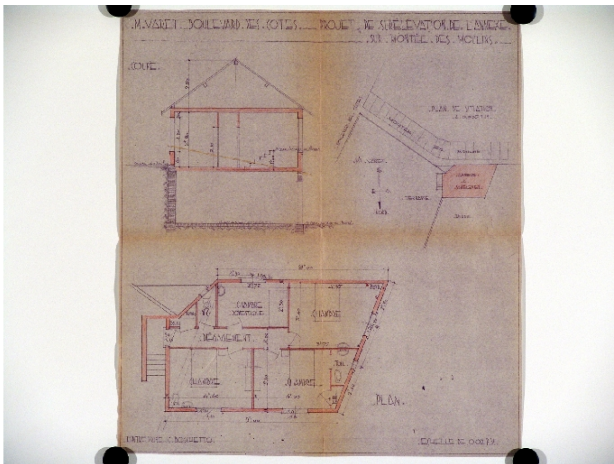
Surélévation : plan et coupe
