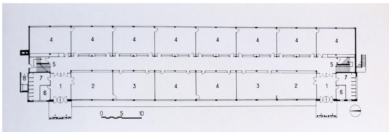
Plan du rez-de-chaussée v. 1961 (Phot. Littoz-Baritel In Noviant, Internat du lycée de garçons, 1963)
