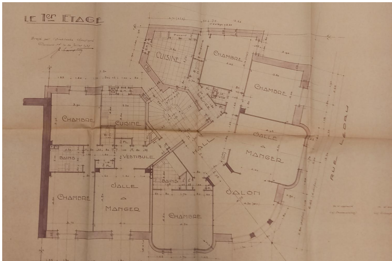
Plan du premier étage. Comparaison 68 boulevard Cote-Blatin
