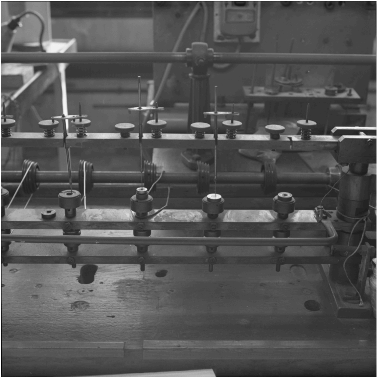
Glacuses (machines à polir le cône).
