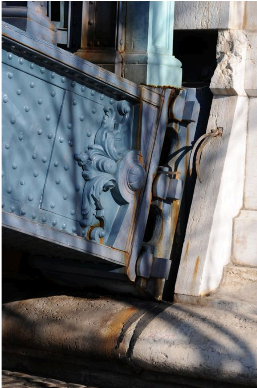
Culée gauche, face aval, vue de détail : ancrage de l'arche (depuis la rive gauche)
