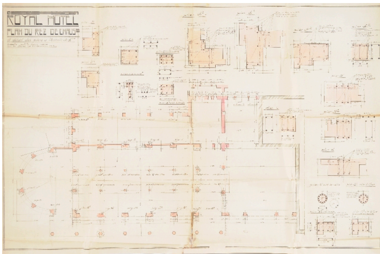
Plan du rez-de-chaussée et détail des piliers
