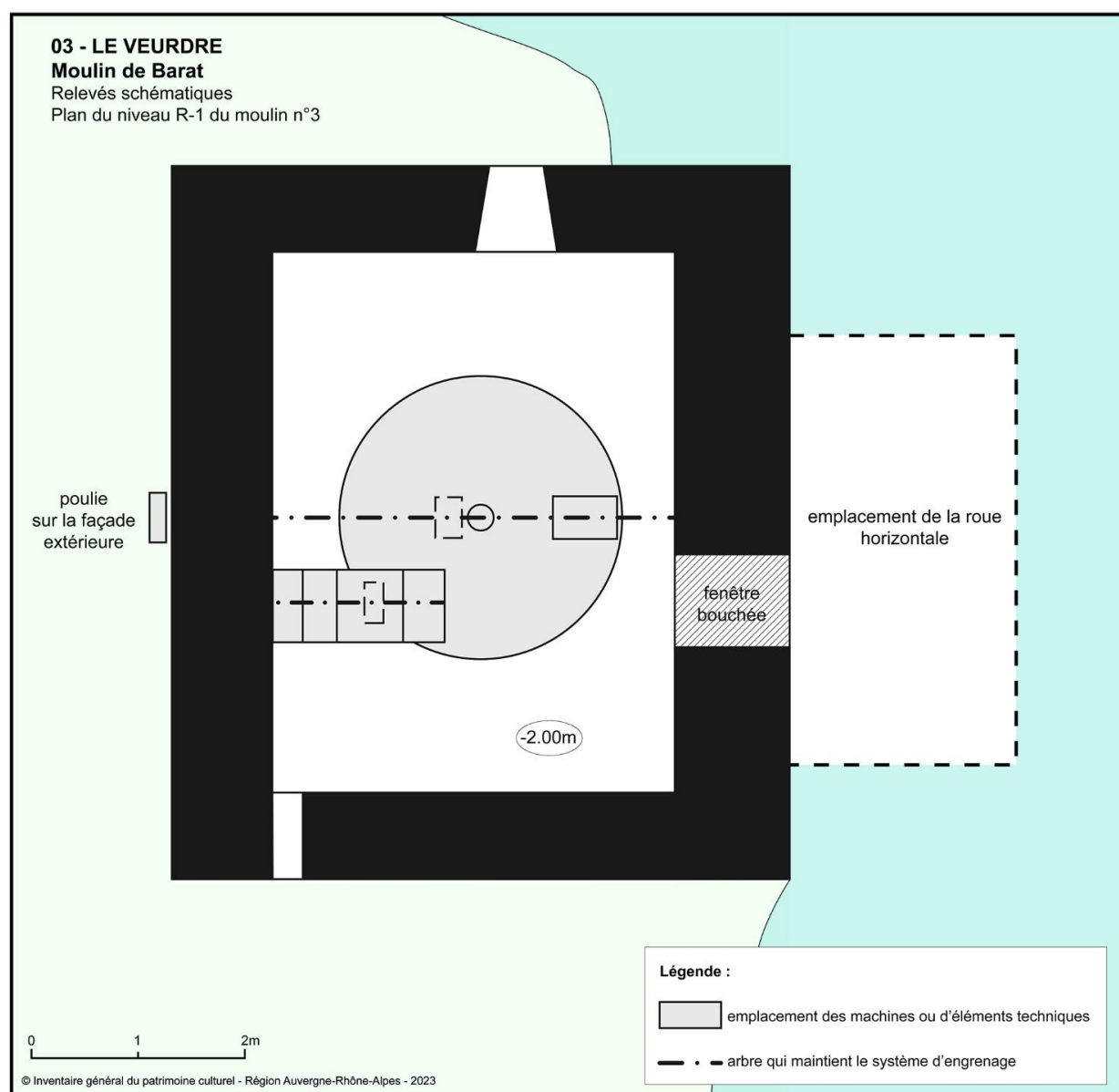
Plan soubassement du moulin 3
