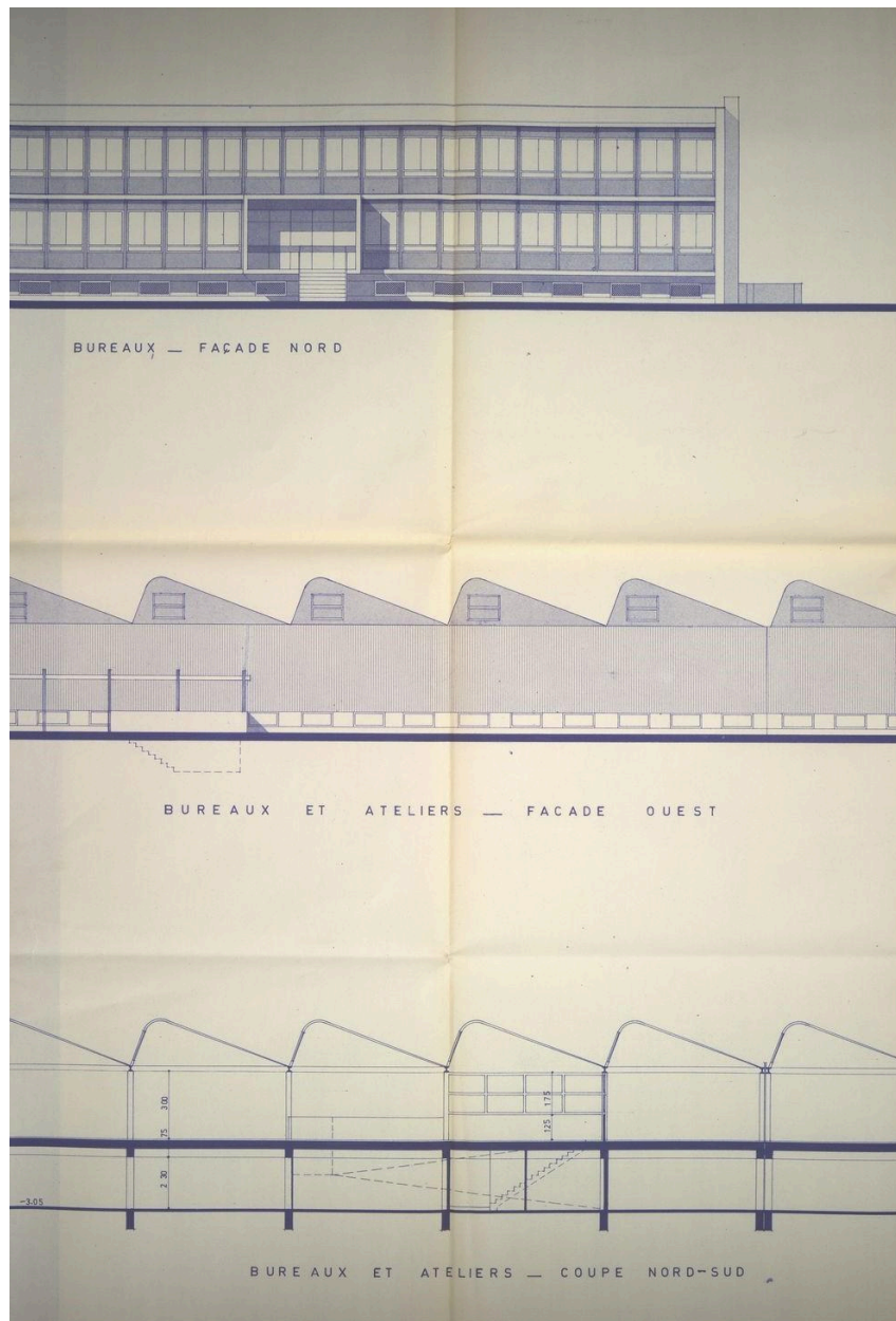
Façade et coupe (AC Villeurbanne, planche 25, 1965)
