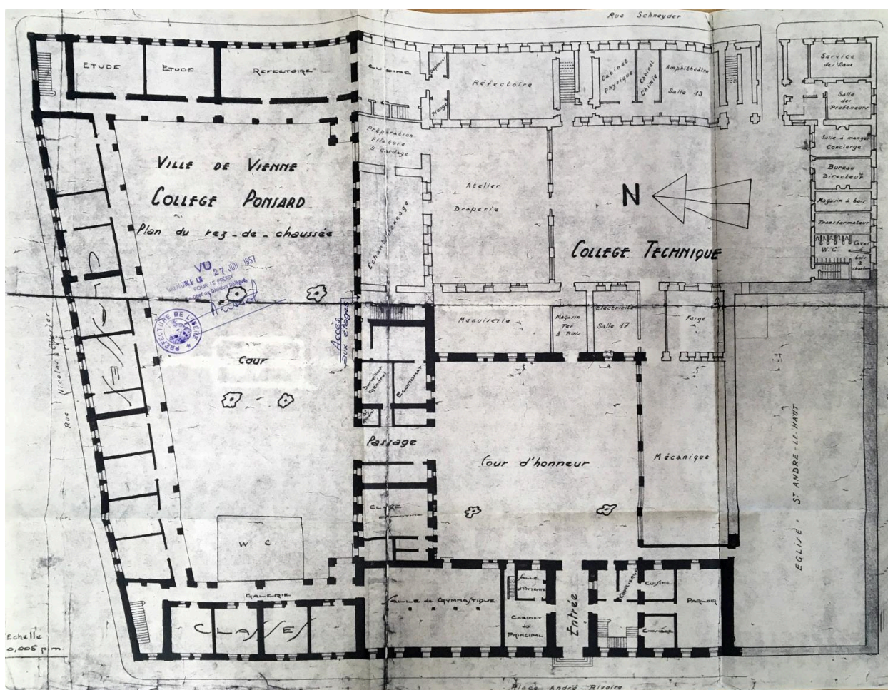
Plan du rez-de-chaussée, état des lieux, 1957 (AD Isère, 5 T 2/26)
