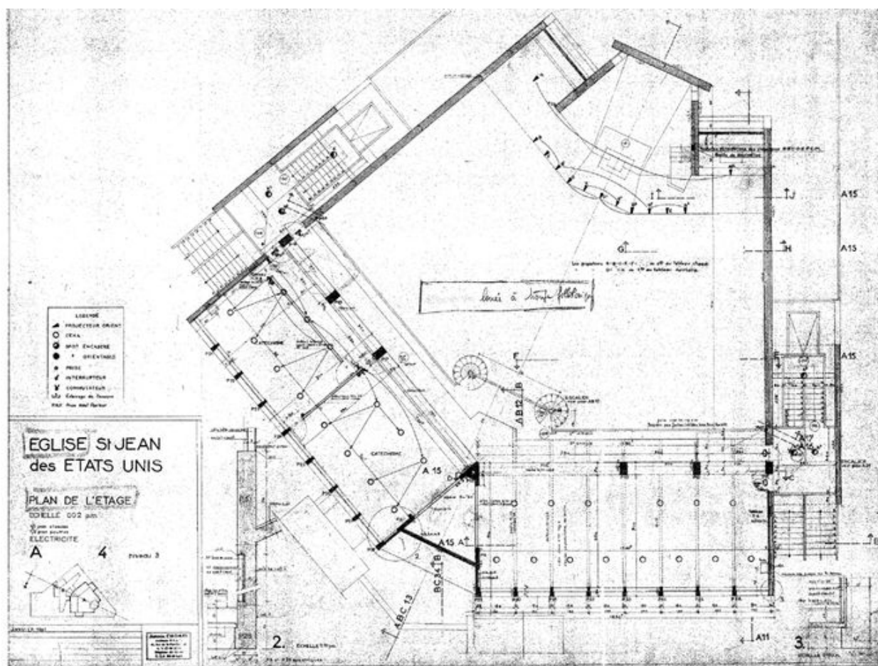
Plan de l'étage de l'église, Alain Chomel, 1961
