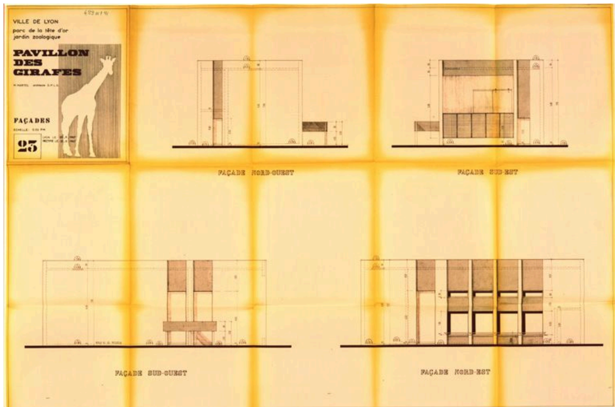
Pavillon des girafes, façades cotées, M. Martel, 1967
