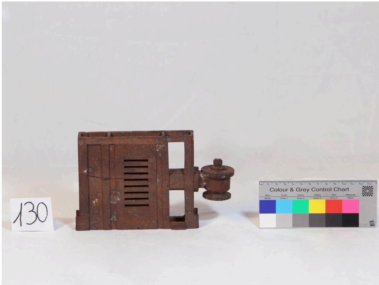
Modèle de hotte aspirante (liste supplémentaire n°130), vue de face
