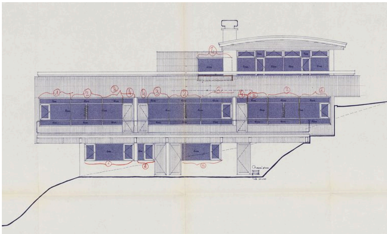
Élévation sud-ouest. Atelier d'Architecture en Montagne, février 1976 (AD Savoie. 6J 1501)
