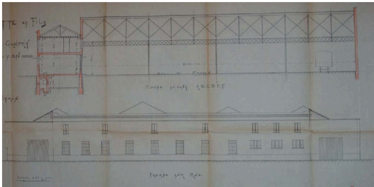
Ets Brossette ; construction de bâtiments ; coupe et façade (1923)
