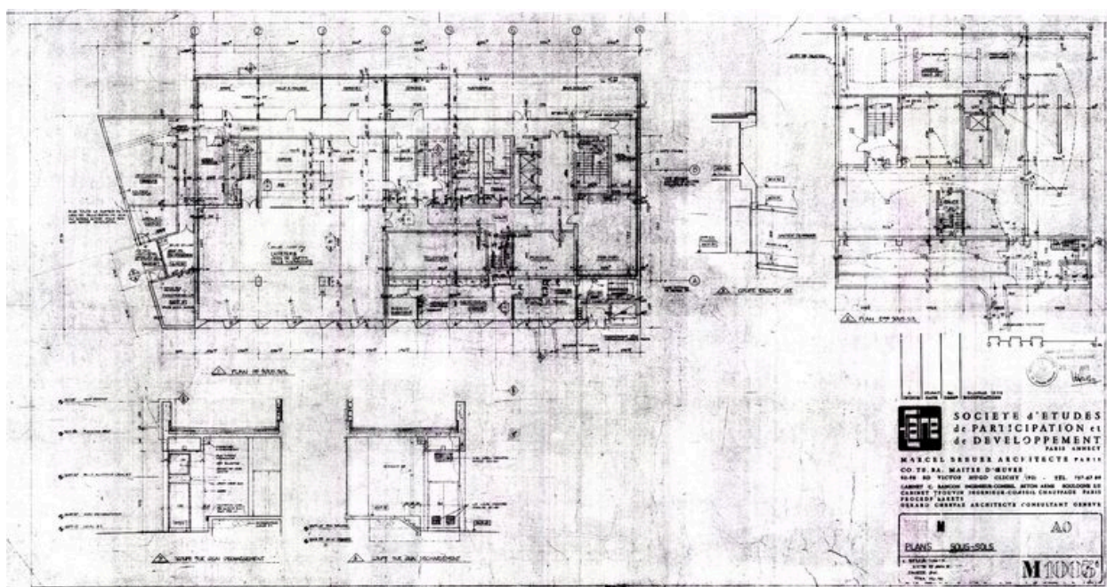
Hôtel M. Plans des sous-sols. Marcel Breuer architecte, 27 janvier 1971. Modifié le 29 janvier 1972 (AC Arâches-la Frasse)
