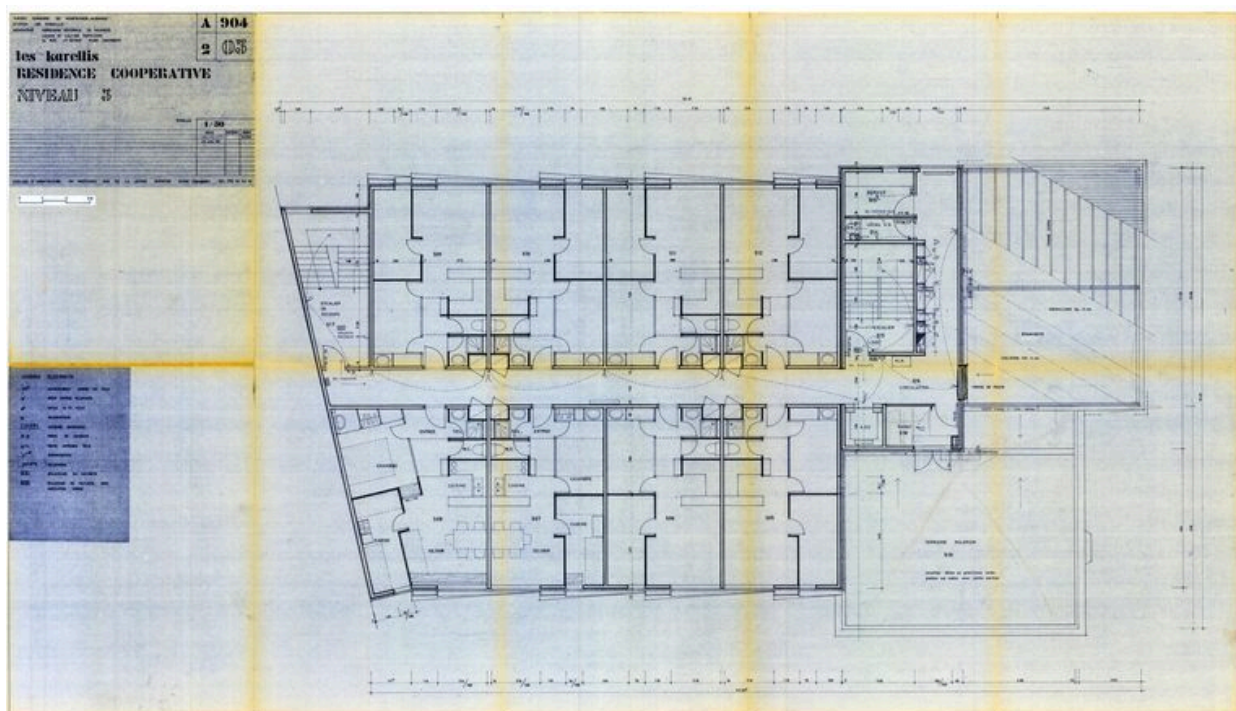
Résidence coopérative. Niveau 5. Plan /Atelier d'architecture en Montagne, Guy Rey-Millet, 13 décembre 1977, 15 février 1978 (AC Montricher-Albanne)
