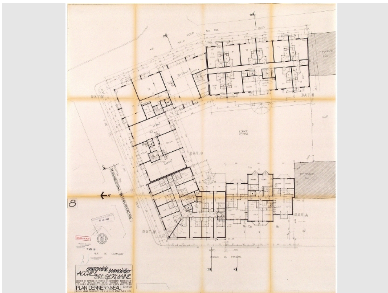
Plan du dernier niveau
