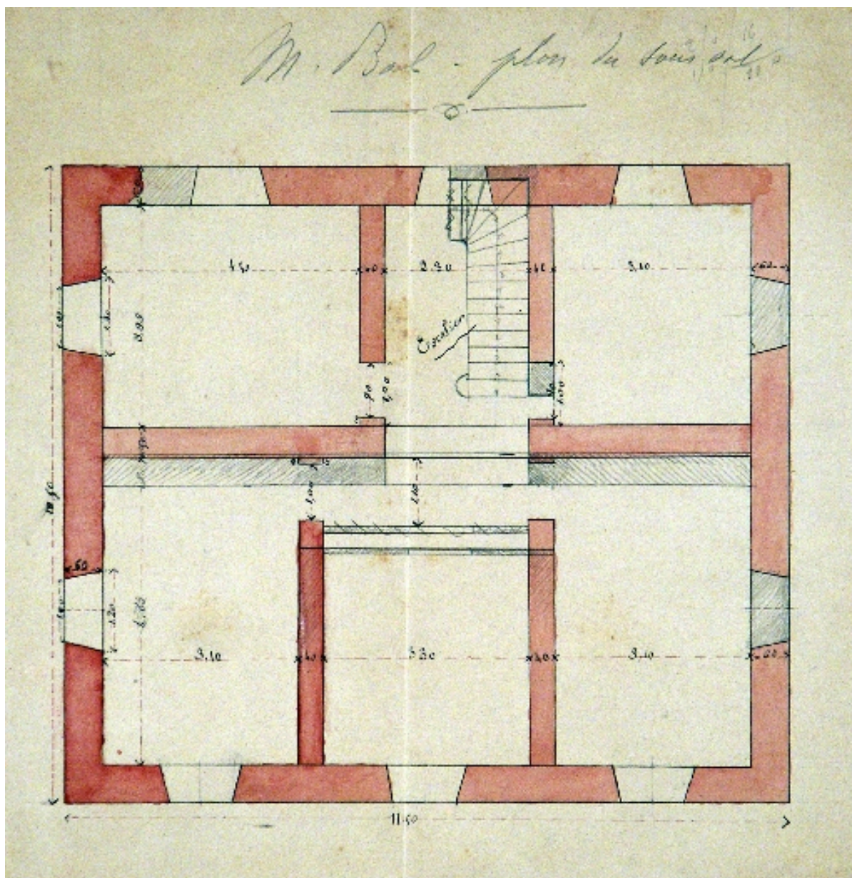
Plan du sous-sol
