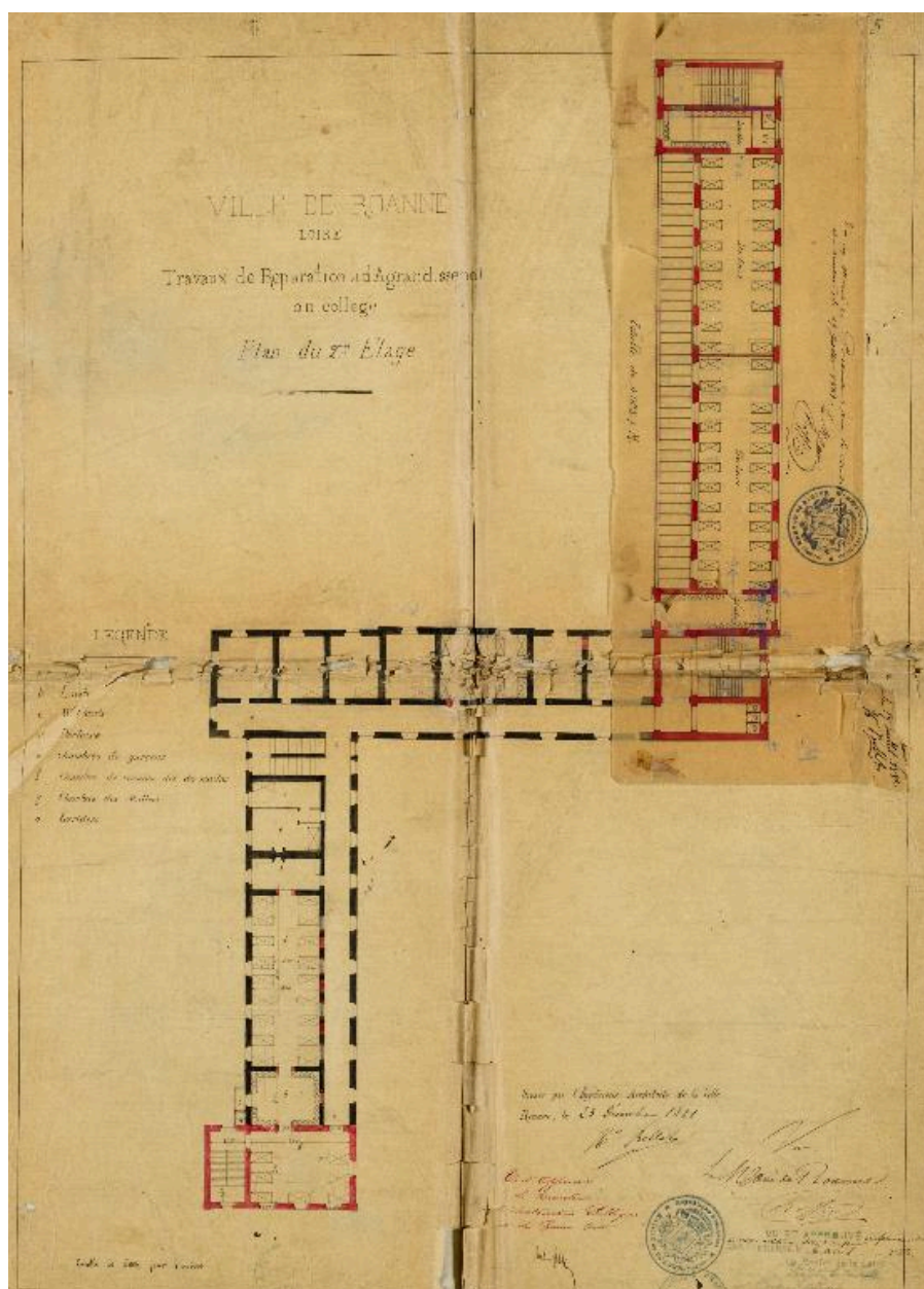
Travaux de réparation et d'agrandissement du collège / plan du 2ème étage / feuille N°3. Bellet (23 décembre 1881)
