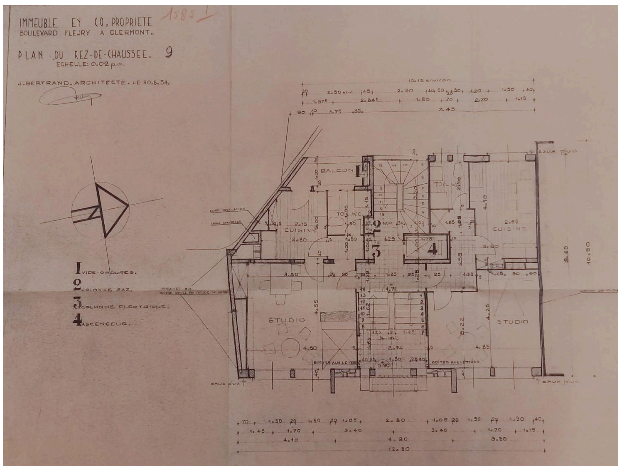
Plan du rez-de-chaussée (1954)
