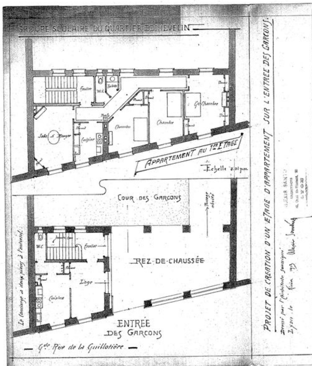
Plan d'un projet d'aménagement d'un appartement sur l'entrée de l'école des garçons, 1913
