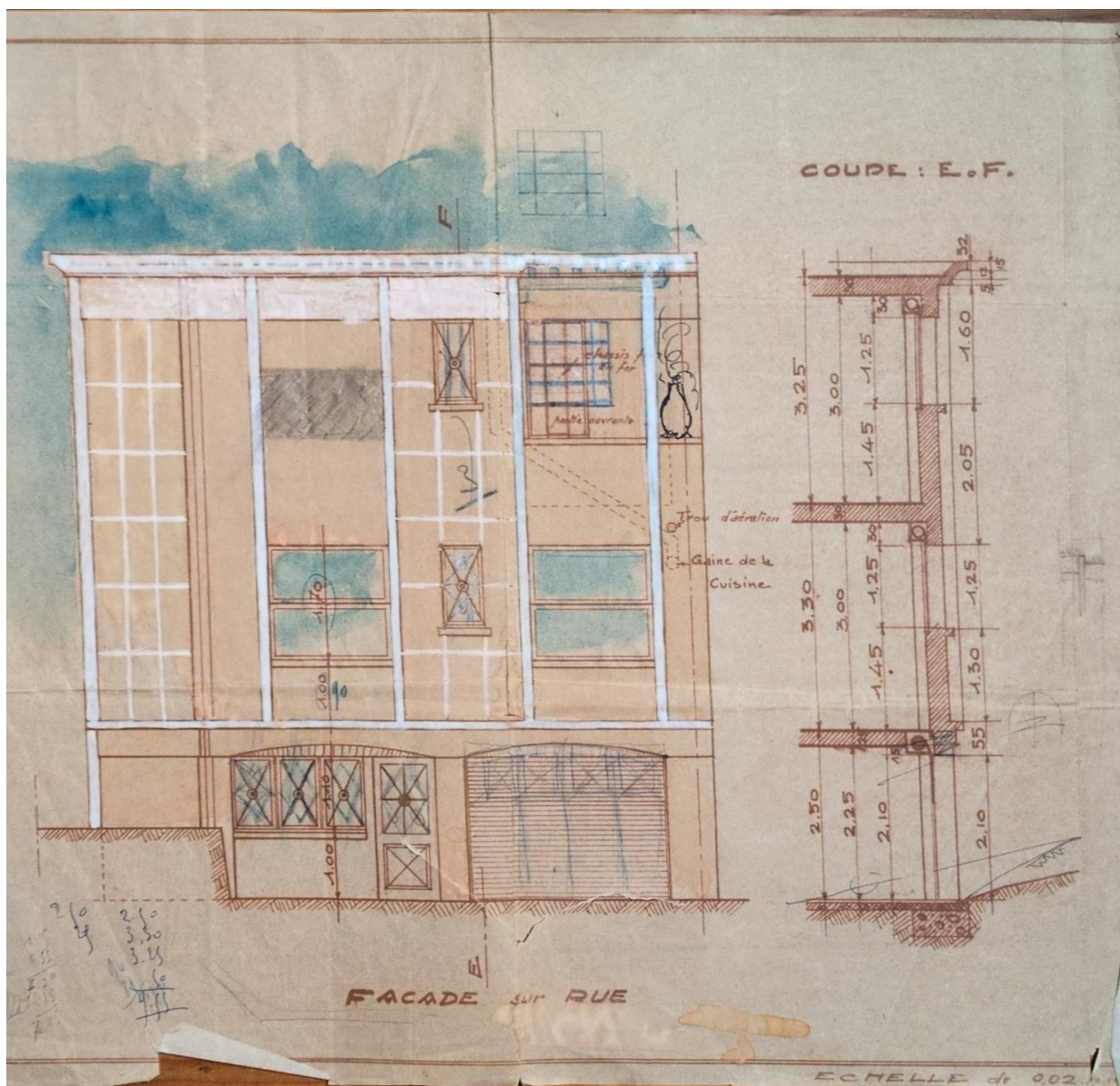
Elévation latérale sur la rue des Prés-Bas (plans modificatifs 1934)
