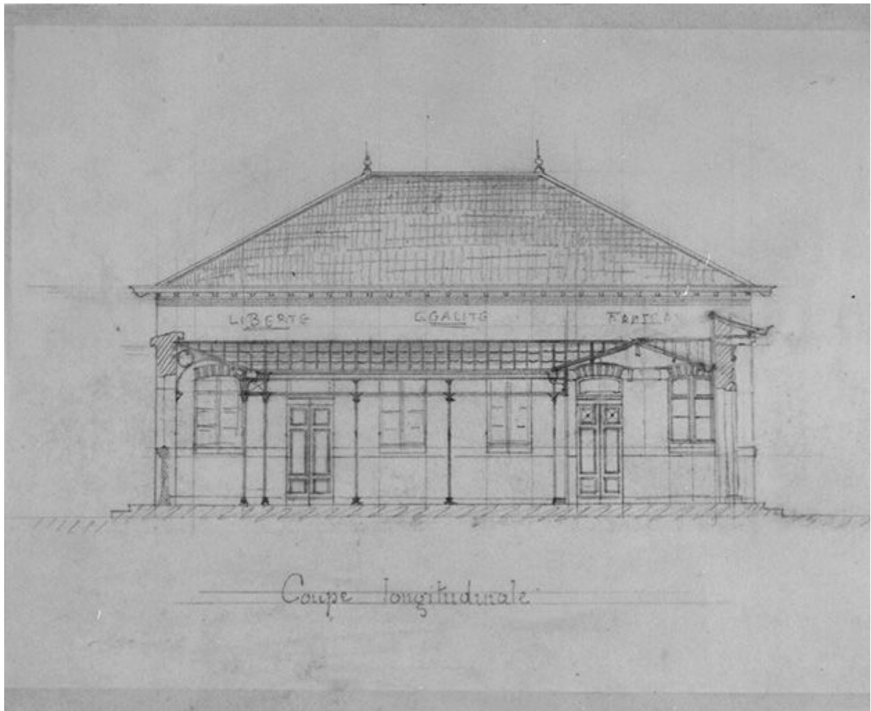
Coupe longitudinale
