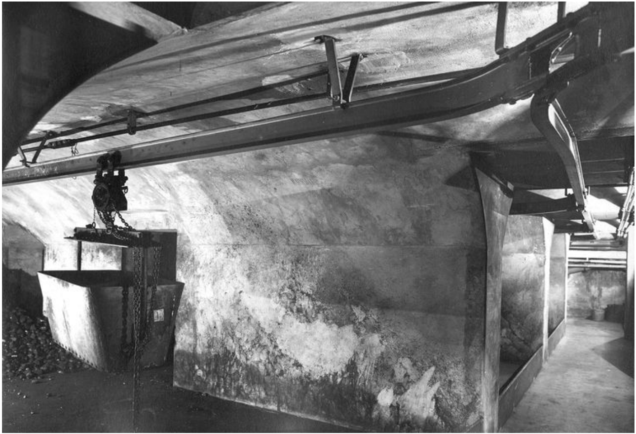
Vue du système de transport du charbon dans les sous-sols (Banque de France, PHAR, non coté, photographie).
