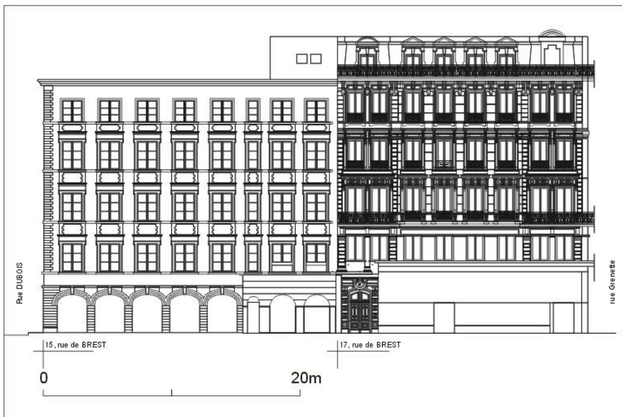
Elévation du côté est de la rue de Brest, détail entre la rue Dubois et la rue Grenette, d'après un relevé photogrammétrique par A. Bensaci, 2003
