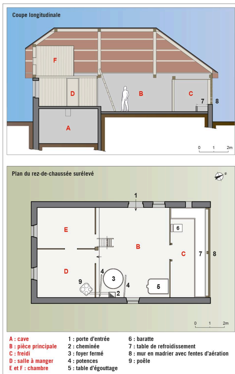
Plan du rez-de-chaussée surélevé et coupe longitudinale (fond : relevé André Céréza)
