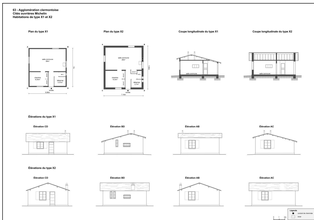
Plan des habitations de types X1 et X2.
