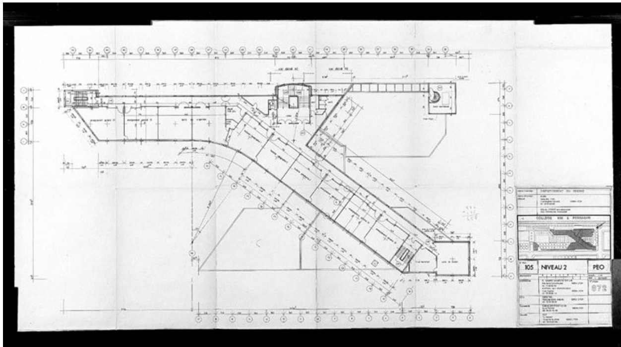
Plan du deuxième étage carré
