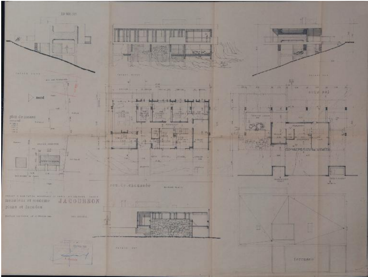
Villa non réalisée : plans et façades, 1965
