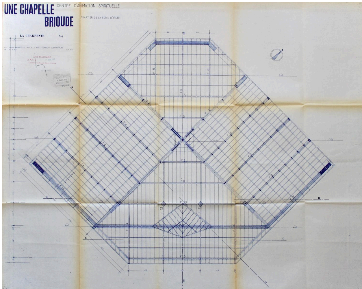
Brioude, chapelle de la Borie Darles, plan de la charpente (projet non définitif), 30 mars 1965, Guy Bion architecte, Archives de la paroisse Saint-Julien de Brioude.
